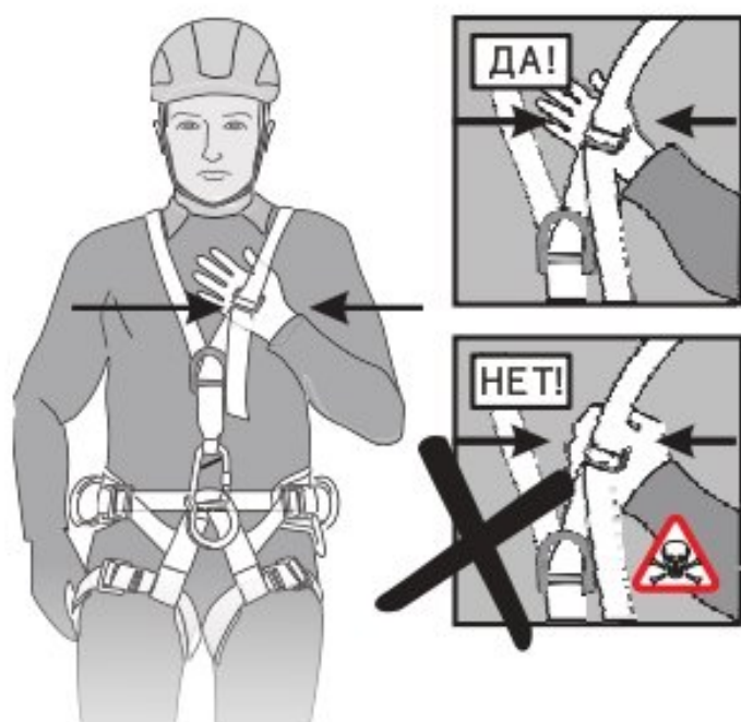
Рис. 8. Натяжение лямок привязи
