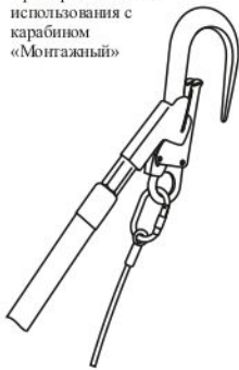
Рис. 3. Последовательность инсталляции страховочной системы
