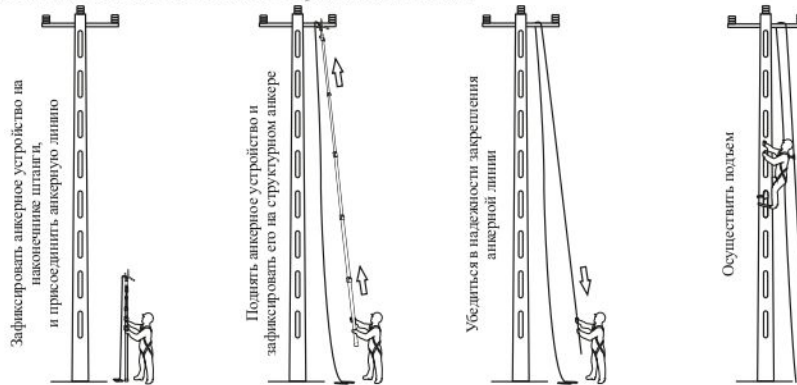
Рис. 3. Последовательность инсталляции страховочной системы
